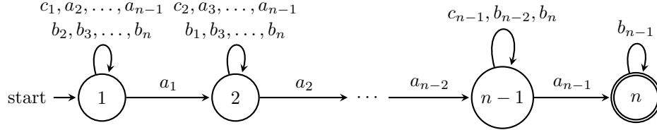
Fig. 1. The DFA A_n
