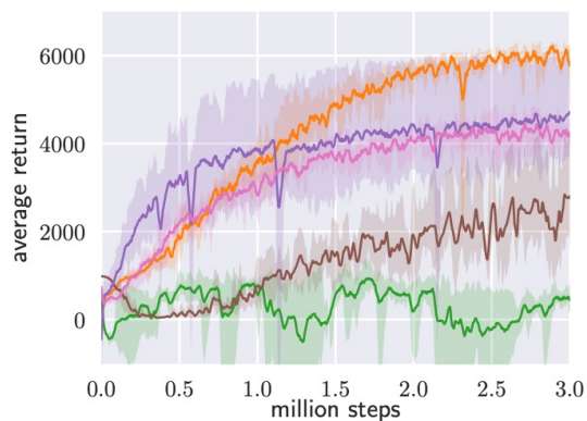
(d) Ant-v1
