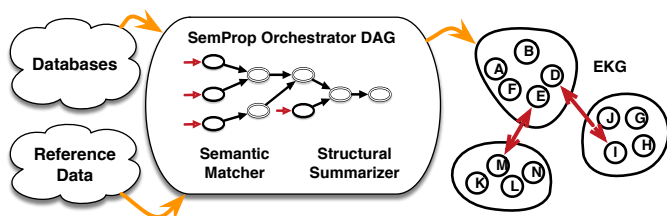
Fig. 2: SemProp overview
